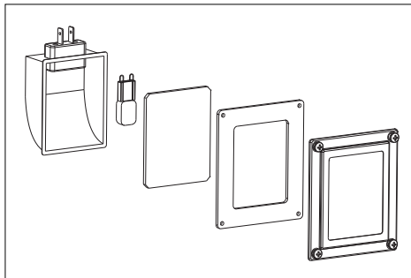
Oświetlenie piekarnika
