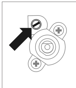
Regulacja zaworu DEFENDI z zabezpieczeniem przeciwwypływowym
