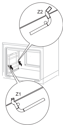
Demontaż drabinek bocznych
