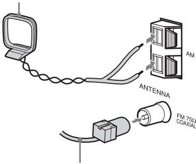
AM-kaderantenne
